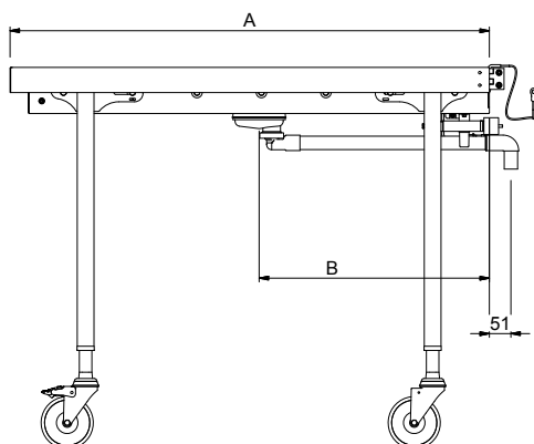
Front aanzicht
